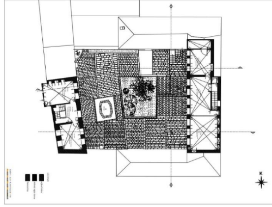
Şekil 6. Üzeyir BeyKonağı 1. kat planı (Çalın, vd., 2015).
