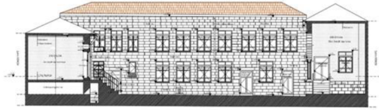
Şekil 10. Konağın doğu cephesini gösteren kesit (Çalın vd., 2015).
