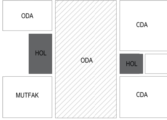
Şekil 6.2. İki Sirkülasyon Mekanının Dışında Yaşam Alanının da Geçiş Mekânı Olduğu Plan Şeması
