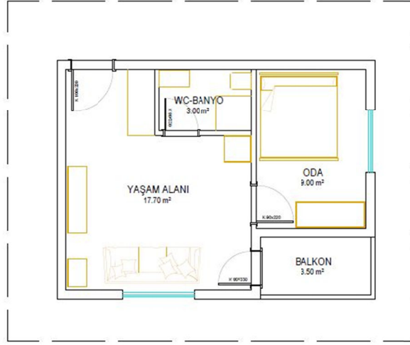
Şekil 5.11. Özçil Rezidans Daire Planı (Dairenin rölövesi alınıp yeniden çizilmiştir.)
