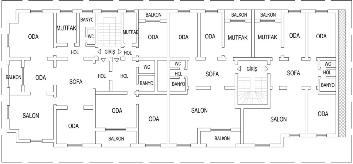
Şekil 4.6. Abdulkadir Göksel Apartmanı Kat Planı (Erbalçı, 2021’den yeniden çizilmiştir.)
