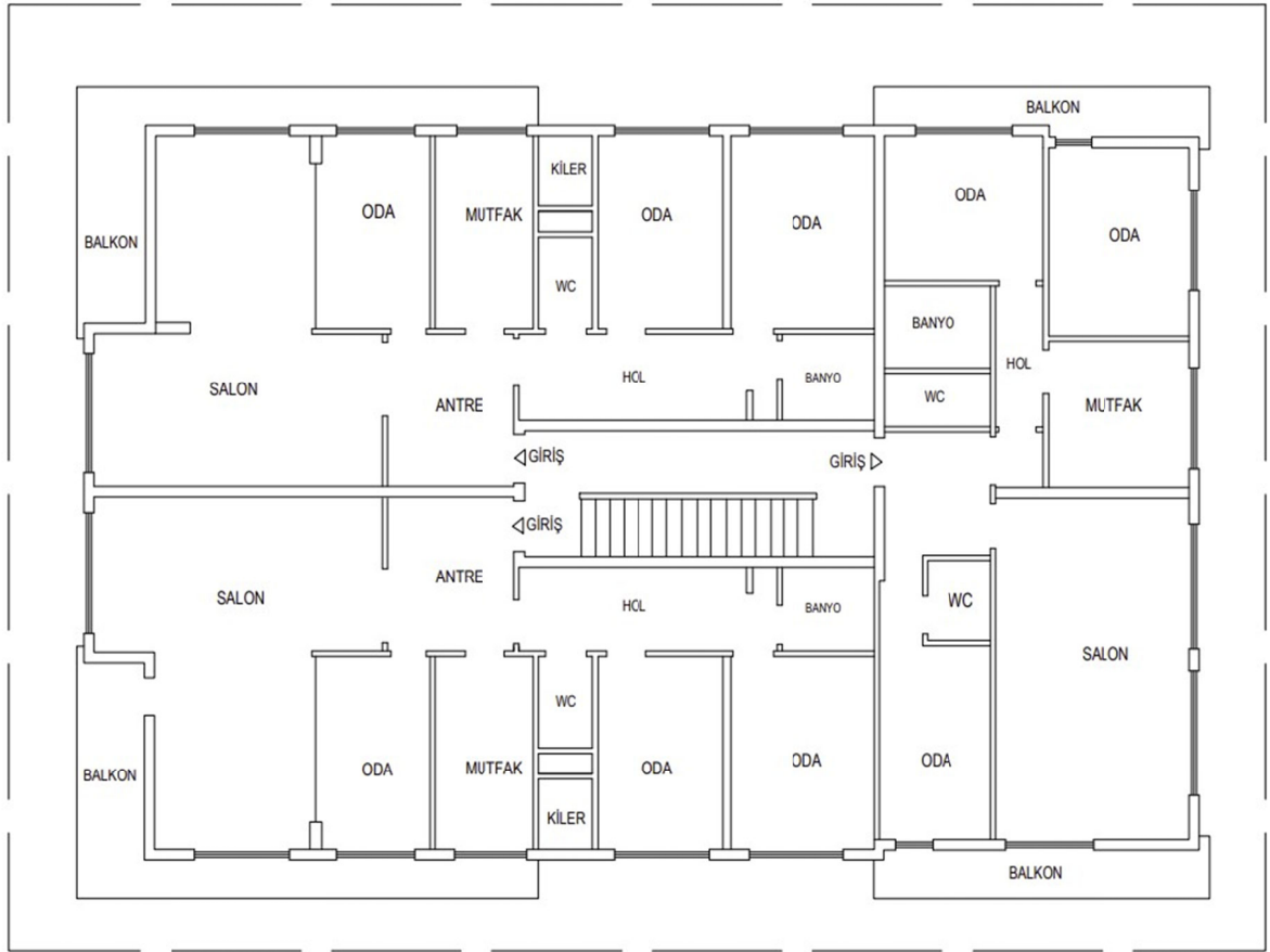
Őekil 4.19. Bahar Apartmanı Normal Kat Planı (Őahin, 2022’den yeniden  izilmiŐtir.)
