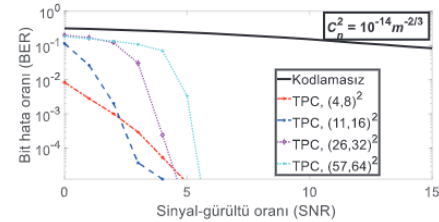
Şekil 4: Orta türbülansta genişletilmiş hamming kod tabanlı TPC’nin BER performansı.
