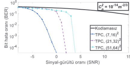
Şekil 6: Orta türbülansta genişletilmiş BCH kod tabanlı TPC’nin BER performansı.
