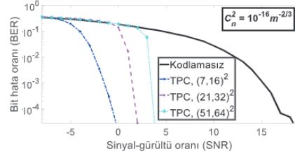
Şekil 5: Zayıf türbülans genişletilmiş BCH kod tabanlı TPC’nin BER performansı.
