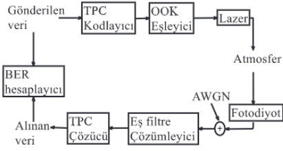
Şekil 2: Tasarlanan optik haberleşme sisteminin blok şeması
