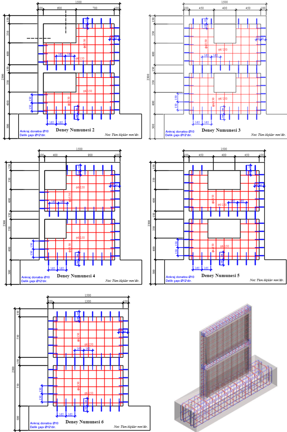
Şekil 3. Güçlendirilmiş numunelerin boyut ve donatı detayları Figure 3. Details of dimensional and reinforcement of strengthened specimens
