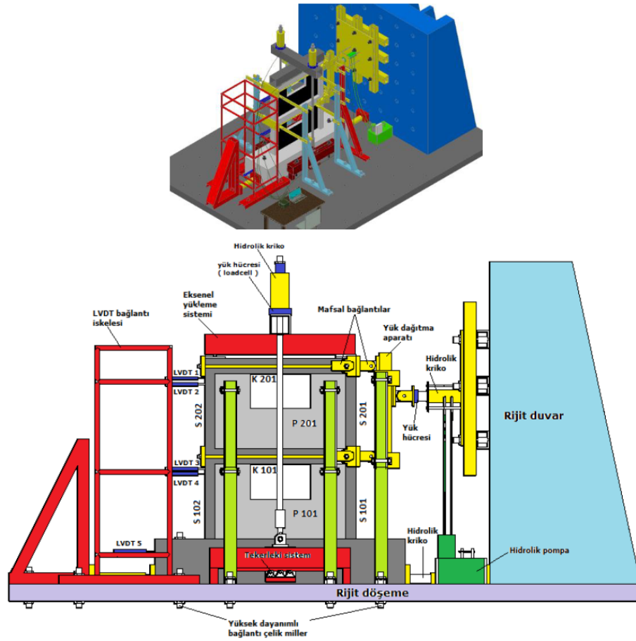
Şekil 4. Yükleme düzenegi
