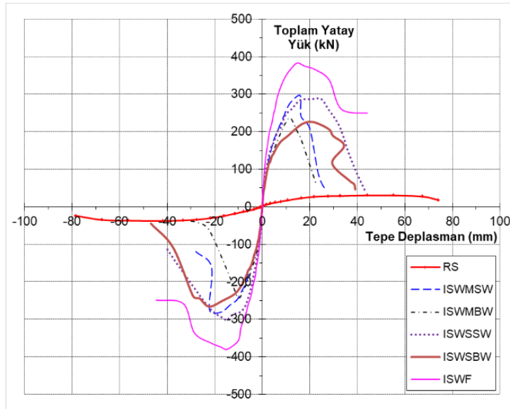
Şekil 17. Deney numunelerinin zarf eğrileri
