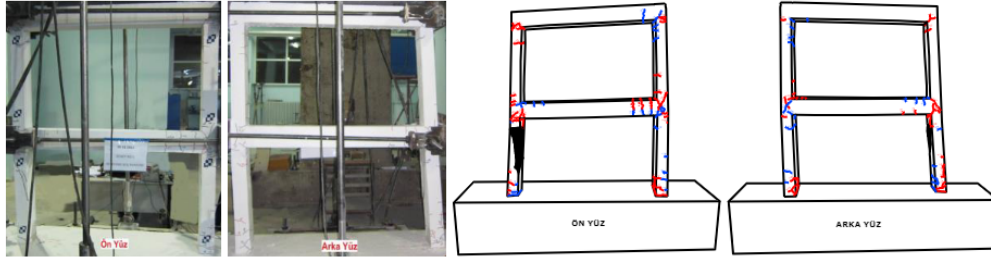
Şekil 5. Deney sonrası, Deney Numunesi 1 (RS)'nin görünümü
