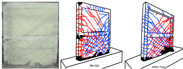
Şekil 15. Deney sonrası, Deney Numunesi 6 (ISWF)’nin görüntüsü
