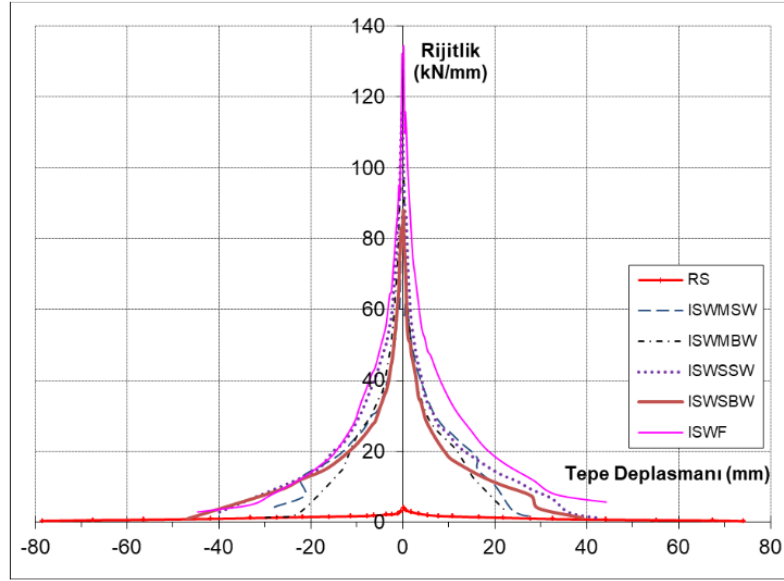
Şekil 18. Deney numunelerinin rijitlik eğrileri
