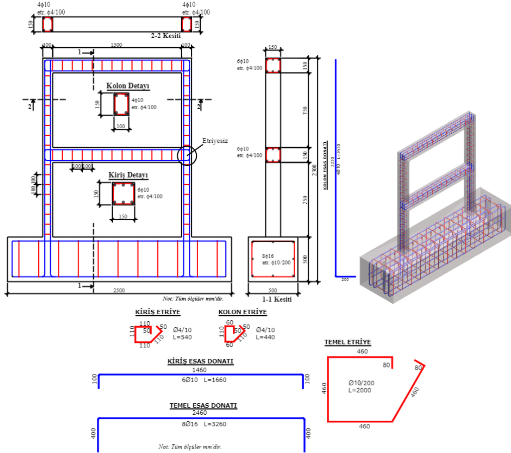
Şekil 1. Betonarme çerçevelerin boyut ve donatı detayları
