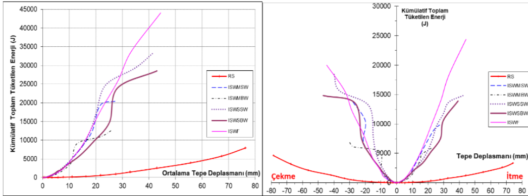
Şekil 19. Deney numunelerine ait enerji tüketimi eğrileri
