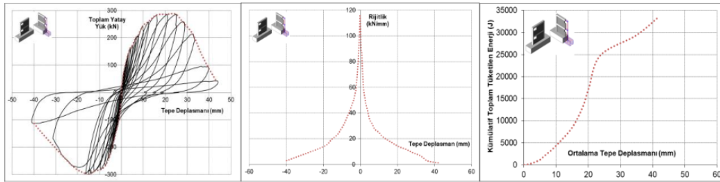
Şekil 12. Çevrimsel histeresis, dayanım zarfı, rijitlik ve enerji tüketimi eğrileri (Deney Numunesi 4) Figure 12. Cyclic hysteresis, envelopes, stiffness and energy dissipation curves (Specimen 4)
