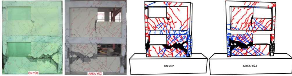
Şekil 7. Deney sonrası, Deney Numunesi 2 (ISWSBW)'nin görünümü
