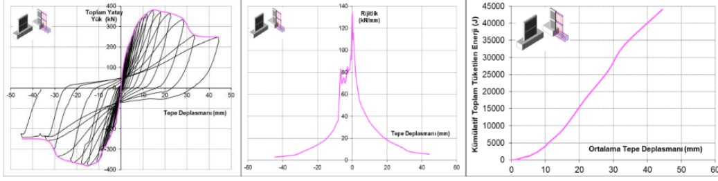
Şekil 16. Çevrimsel histeresis, dayanım zarfı, rijitlik ve enerji tüketimi eğrileri (Deney Numunesi 6)
