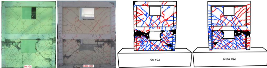
Şekil 9. Deney sonrası, Deney Numunesi 3 (ISWMSW)'nin görünümü
