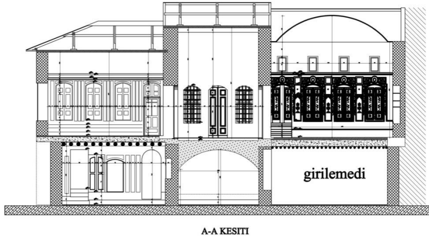
Şekil 8. 233. Guertasirats Okulu'nun Son Binası Nicholas Nazaretyan'ın Evi A-A Kesiti (Gaziantep Kudeb Arşivi, 2019)
