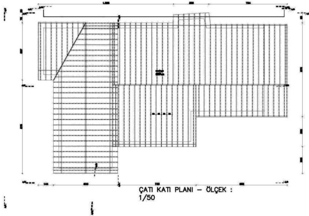
Şekil 8. 213. Hayganuşyan Kız Lisesi Çatı Katı Planı (Gaziantep Kudeb Arşivi, 2019)
