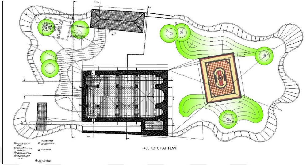
Şekil 8. 36. Ömer Ersoy Kültür Merkezi +436 Kotu Kat Planı Restorasyon Sonrası (Gaziantep Kudeb Arşivi, 2019)
