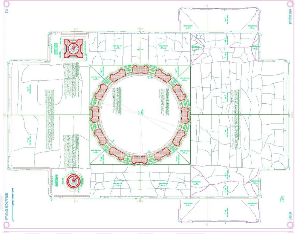
Şekil 8. 77. Kurtuluş Cami Zemin Kat +20303 Kotu Planı Rölöve (Gaziantep Kudeb Arşivi, 2019)
