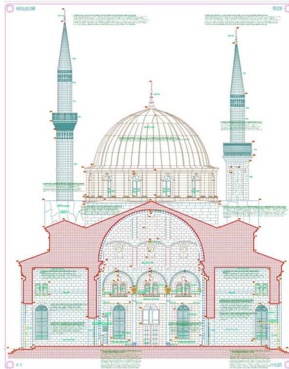
Şekil 8. 80. Kurtuluş Cami F-F Kesiti Rölöve (Gaziantep Kudeb Arşivi, 2019)
