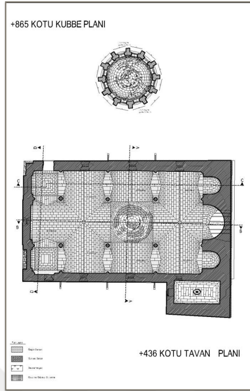
Şekil 8. 28. +436 Kotu Tavan Planı ve +865 Kotu Kubbe Planı Restorasyon Öncesi Rölöve (Gaziantep Kudeb Arşivi,2019)
