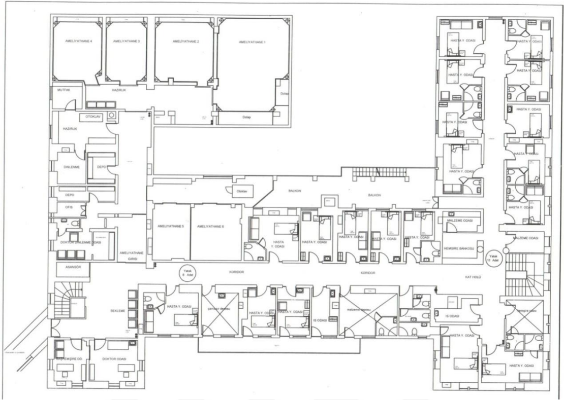
Şekil 8. 180. Amerikan Hastanesi Yataklı Servis 1. Kat Planı Restorasyon Sonrası 2007 (A. Uğraş Arşivi, 2019)
