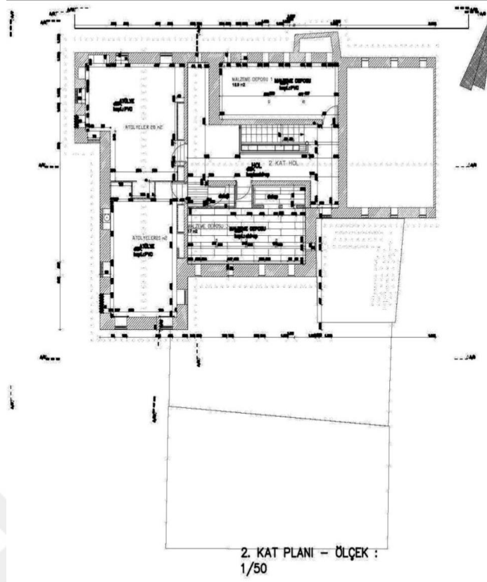
Şekil 8. 209. Hayganuşyan Kız Lisesi 2. Kat Planı (Gaziantep Kudeb Arşivi, 2019)
