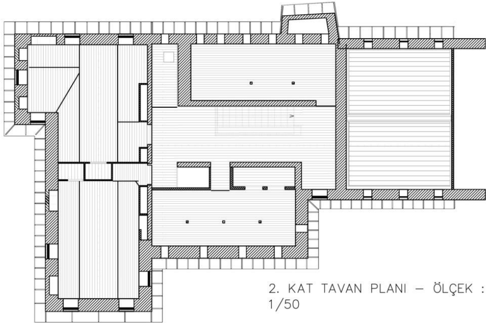
Şekil 8. 210. Hayganuşyan Kız Lisesi 2. Kat Tavan Planı (Gaziantep Kudeb Arşivi, 2019)
