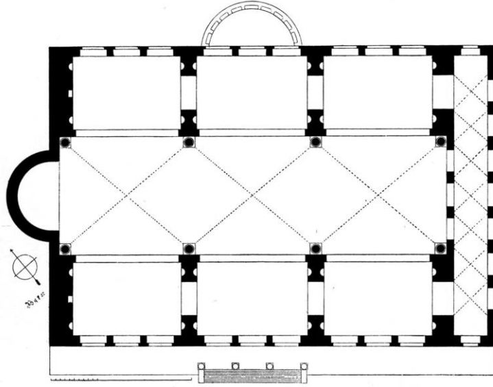
Şekil 7. 2. Roma Bazilika Planı (Maxentius Basilica, Rome)
