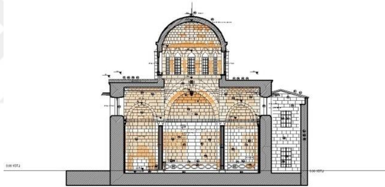
A - A KESİTİ Ö : 1 / 50
