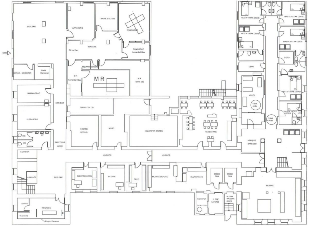
Şekil 8. 179. Amerikan Hastanesi Yataklı Servis Bodrum Kat Planı Restorasyon Sonrası 2007 (A. Uğraş Arşivi, 2019)
