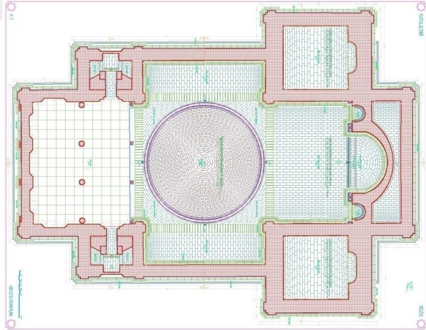
Şekil 8. 76. Kurtuluş Cami -300Kotu Tavan Planı Rölöve (Gaziantep Kudeb Arşivi, 2019)
