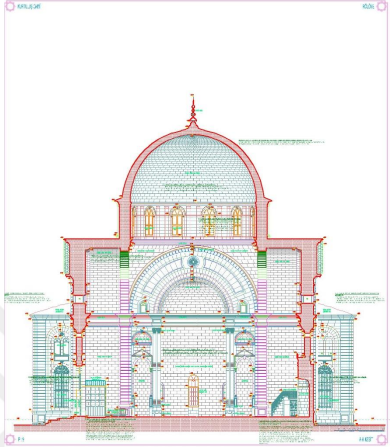
Şekil 8. 78. Kurtuluş Cami A-A Kesiti Rölöve (Gaziantep Kudeb Arşivi, 2019)
