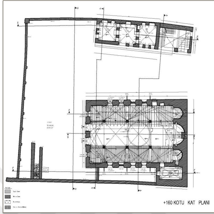
Şekil 8. 27. +160 Kotu Kat Planı Restorasyon Öncesi Rölöve (Gaziantep Kudeb Arşivi, 2019)
