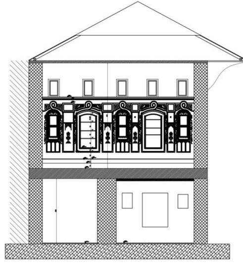
C-C KESİTİ
