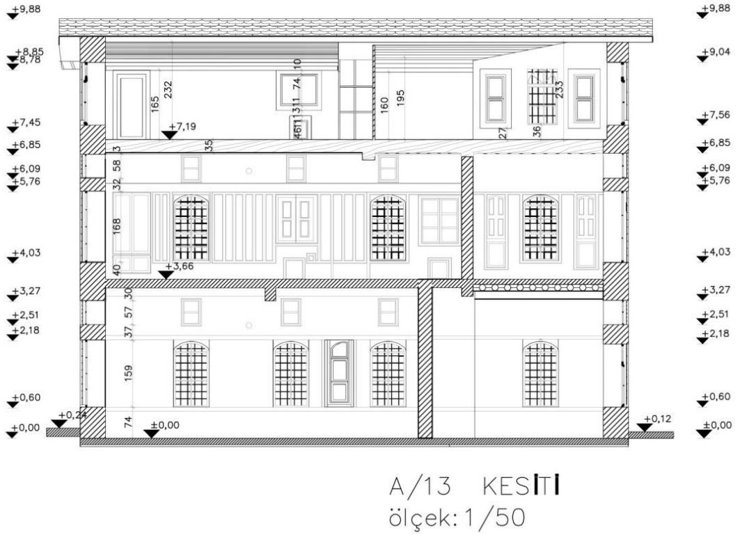
Şekil 8. 214. Hayranuşyan Kız Lisesi A/13 Kesiti (Gaziantep Kudeb Arşivi, 2019)
