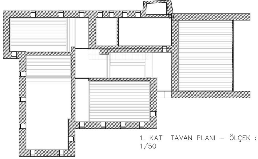
Şekil 8. 211. Hayganuşyan Kız Lisesi 1. Kat Tavan Planı (Gaziantep Kudeb Arşivi, 2019)
