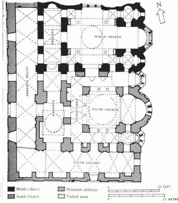
Şekil 7. 4. Kapalı Yunan Haçı Planlı Kilise Planı Alexander Van Millingen, Byzantine Churches of Constantinople, 1912
