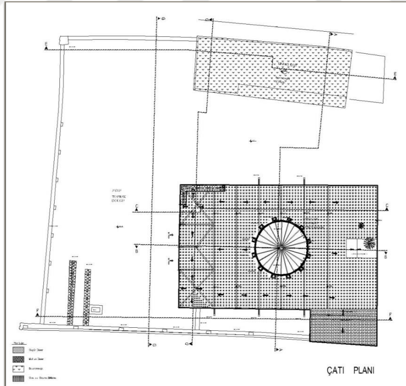
Şekil 8. 29. Çatı Planı Restorasyon Öncesi Rölöve (Gaziantep Kudeb Arşivi,2019)
