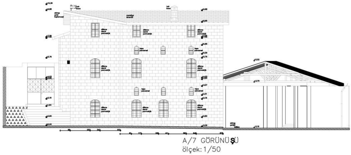
Şekil 8. 216. Hayganuşyan Kız Lisesi A/6 Görünüşü (Gaziantep Kudeb Arşivi, 2019)
