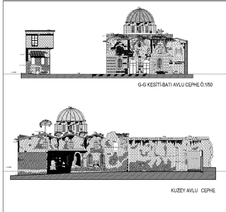
Şekil 8. 32. Aziz Bedros Kilisesi G-G Kesiti Batı Avlu Cephe ve Kuzey Avlu Cephe Restorasyon Öncesi Rölöve (Gaziantep Kudeb Arşivi, 2019)
