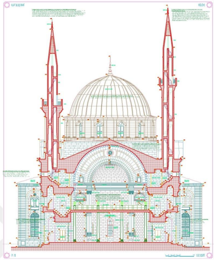
Şekil 8. 81. Kurtuluş Cami E-E Kesiti Rölöve (Gaziantep Kudeb Arşivi, 2019)
