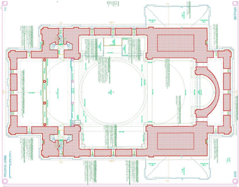
Şekil 8. 75. Kurtuluş Cami Zemin Kat -1221 Kotu Planı Rölöve (Gazinatep Kudeb Arşivi, 2019)
