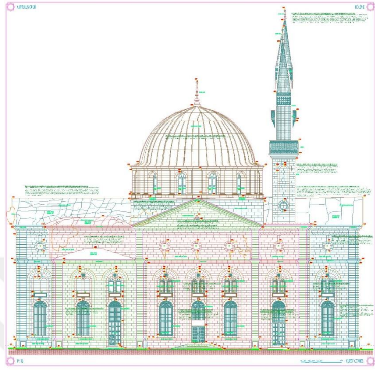
Şekil 8. 82. Kurtuluş Cami Kuzey Cephesi Rölöve (Gaziantep Kudeb Arşivi, 2019)
