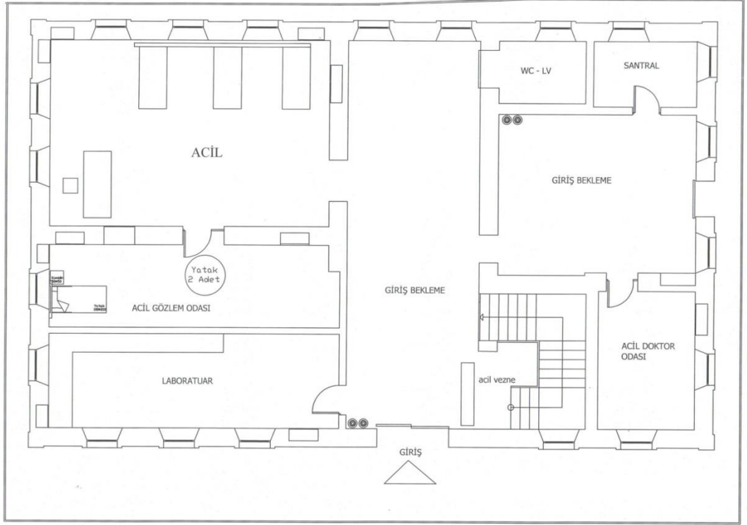
Şekil 8. 175. Amerikan Hastanesi Acil Blok Zemin Kat Restorasyon Öncesi Planı 2001 (A. Uğraş Arşivi, 2019)
