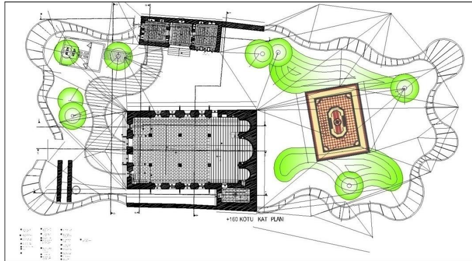
Şekil 8. 34. Ömer Ersoy Kültür Merkezi +160 Kotu Kat Planı Restorasyon Sonrası (Gaziantep Kudeb Arşivi, 2019)
