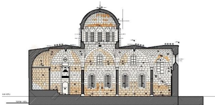
B - B KESİTİ Ö : 1 / 50
