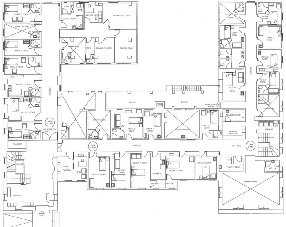
Şekil 8. 178. Amerikan Hastanesi Yataklı Servis Zemin Kat Planı Restorasyon Sonrası 2007 (A. Uğraş Arşivi, 2019)
