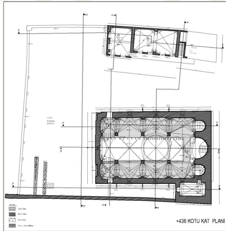
Şekil 8. 26. +436 Kotu Kat Planı Restorasyon Öncesi Rölöve (Gaziantep Kudeb Arşivi, 2019)
