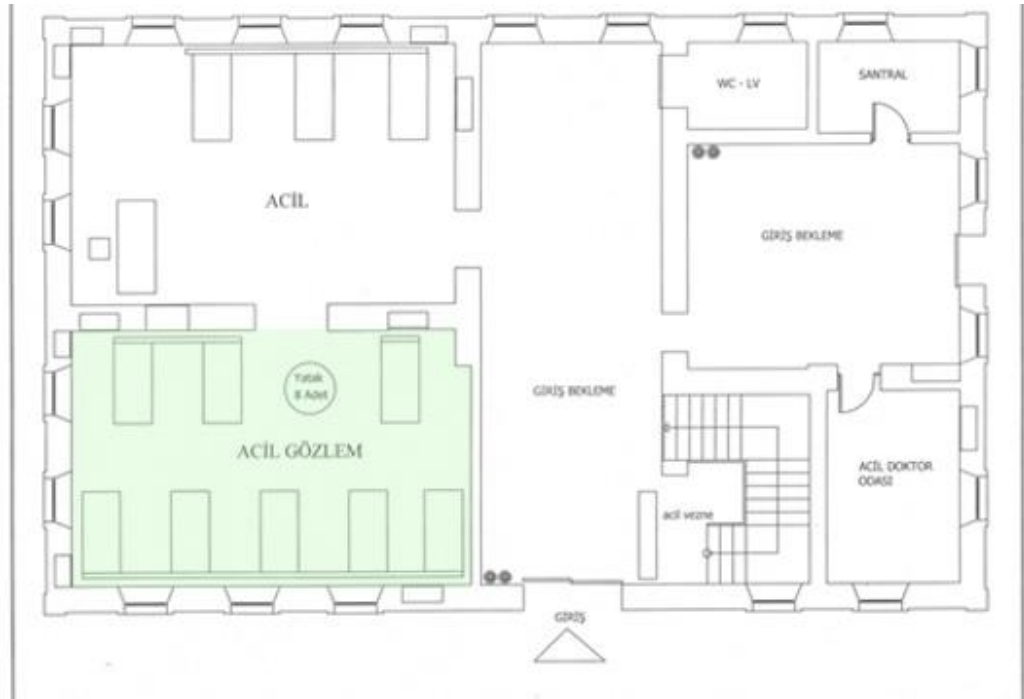
Şekil 8. 174. Amerikan Hastanesi Acil Blok Zemin Kat Restorasyon Sonrası Planı 2007 (A. Uğraş Arşivi, 2019)
