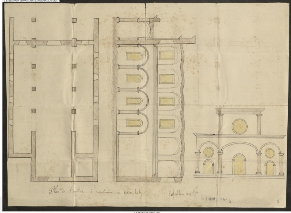
Şekil 8. 60. İlk İnşa Edilen Kendirli Kilisesi 1860 Planı ve Görünüşü (BCA Arşivi, 2019)
