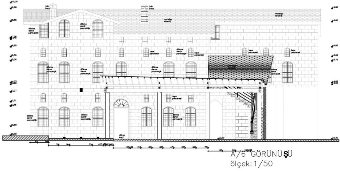
Şekil 8. 217. Hayganuşyan Kız Lisesi A/7 Görünüşü (Gaziantep Kudeb Arşivi, 2019)
