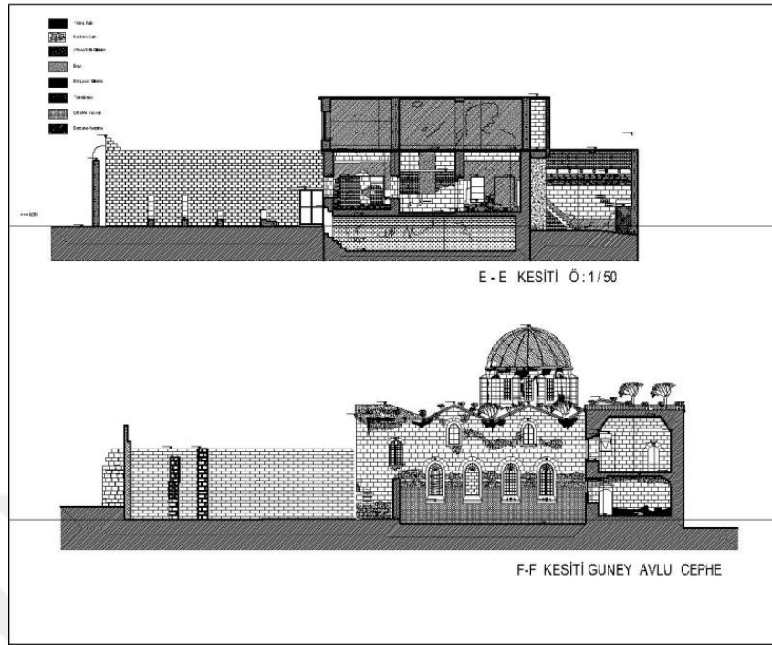
Şekil 8. 33. Aziz Bedros Kilisesi E-E Kesiti ve F-F Kesiti Güney Avlu Cephe Restorasyon Öncesi Rölöve (Gaziantep Kudeb Arşivi, 2019)
