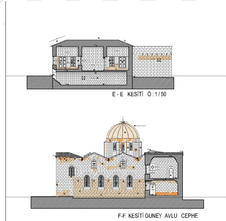
Şekil 8. 40. Ömer Ersoy Kültür Merkezi E-E Kesiti ve F-F Kesiti Güney Avlu Cephe Restorasyon Sonrası (Gaziantep Kudeb Arşivi, 2019)
