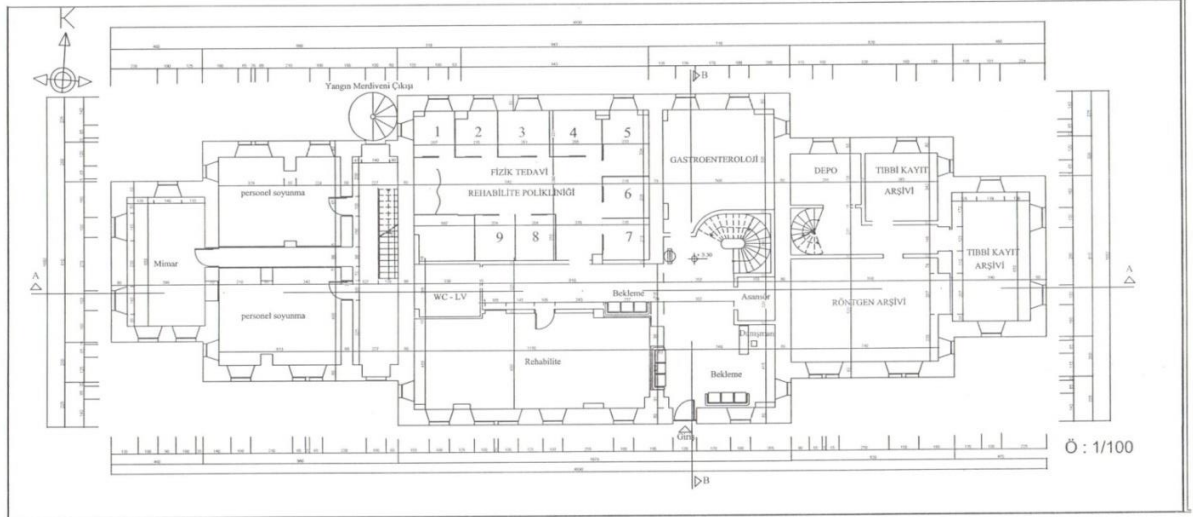
Şekil 8. 185. Amerikan Hastanesi B Blok 1. Kat Planı Restorasyon Sonrası 2007 (A. Uğraş Arşivi, 2019)
