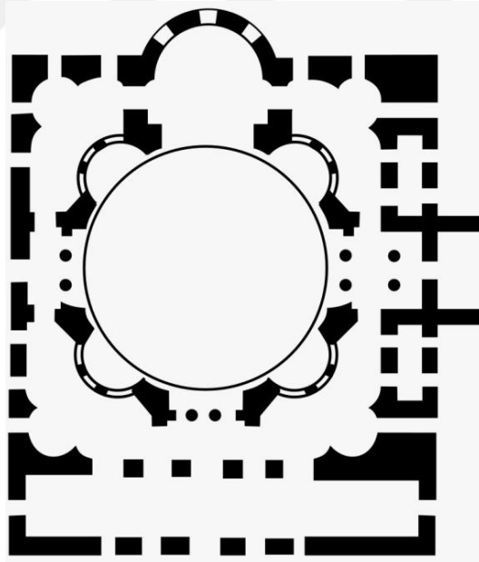
Şekil 7. 5. Merkezi Planlı ve Kubbeli Kilise Planı (Little Hagia Sophia Basilica of San Vitale Constantinople Sergius and Bacchas)
