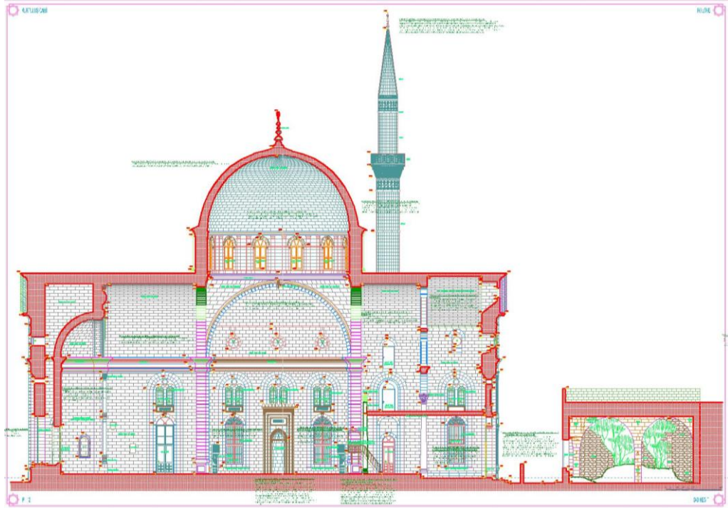
Şekil 8. 79. Kurtuluş Cami D-D Kesiti Rölöve (Gaziantep Kudeb Arşivi, 2019)
