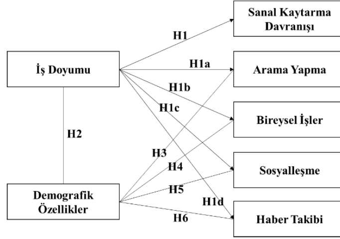
Şekil 1. Araştırma Modeli
